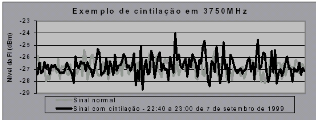
Figura 2.4 – Exemplo de cintilação em sinais de frequência 3,75 GHz, obtido entre as 22 h 40 min e 23 h do dia 7 de setembro de 1999.
