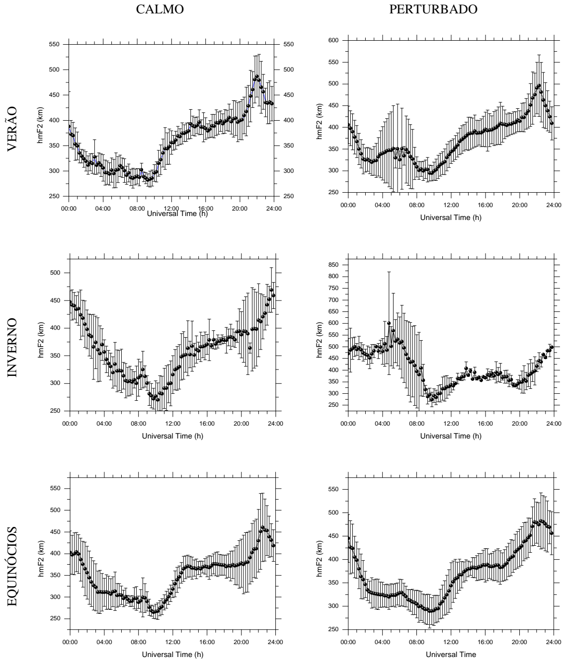
Figura 4.2- Variação da altura média do pico da camada F em relação ao tempo para os períodos calmo e perturbado, nas estações do ano analisadas, obtidos a partir de dados de digissonda no sítio de São Luís- MA.
